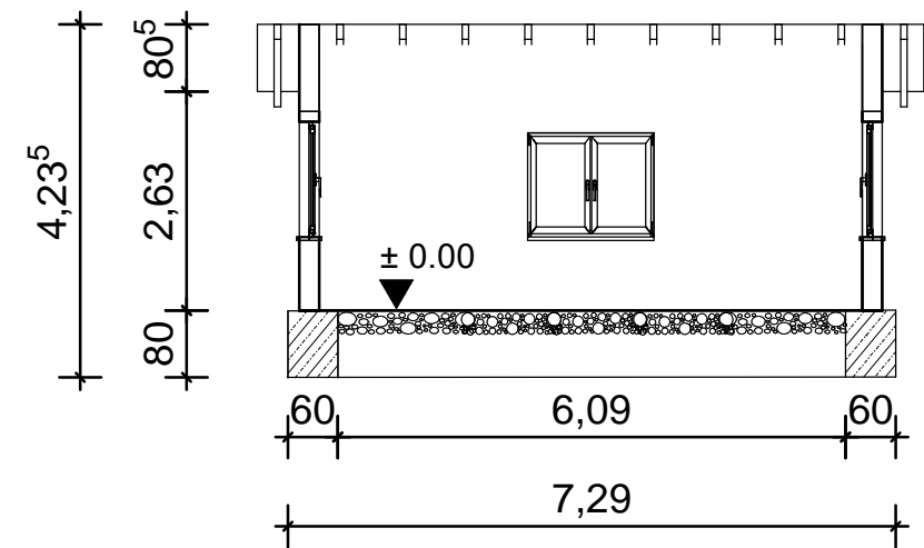
Schnitt A-A
