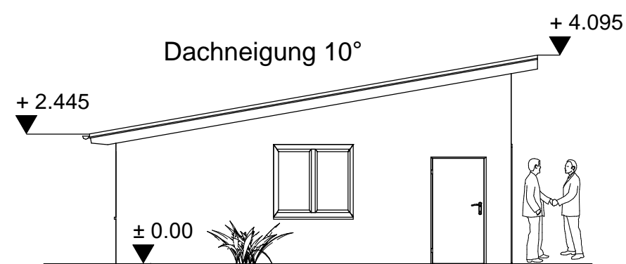
Ostansicht
