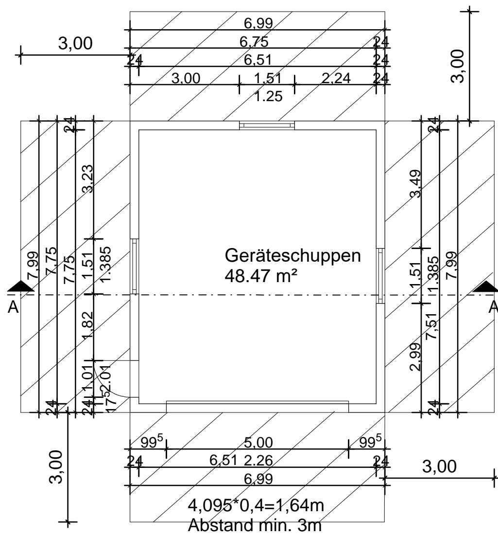
EG
